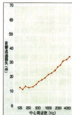
■音響透過損失
